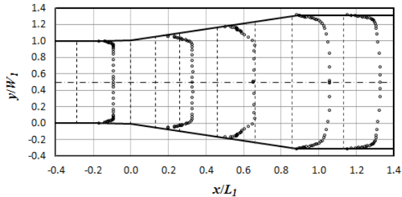
Gambar 2. Distribusi profil kecepatan U/U_{max} pada Re_{Dh} = 1.98 \times 10^5 .
