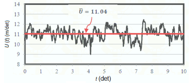
Gambar 9. Fluktuasi kecepatan sebagai fungsi waktu pada outlet elbow kecil.
