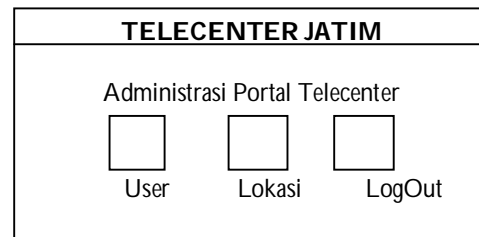
Gambar 9. Rancangan Interface
